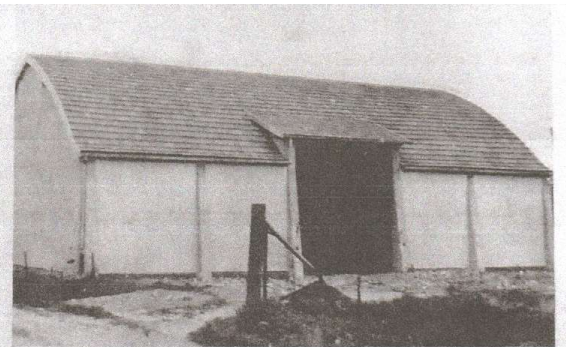
Grange agricole Corbeau, à Epehy (Somme) sur piliers en béton, sans tirants.
