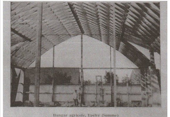
Hangar agricole, Epehy (Somme)
